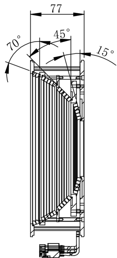
剖面 C-C
