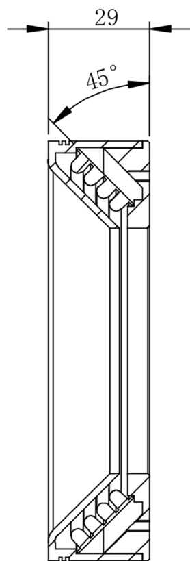
剖面 F-F
